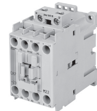
CA7-23E-M22-24E contactor
